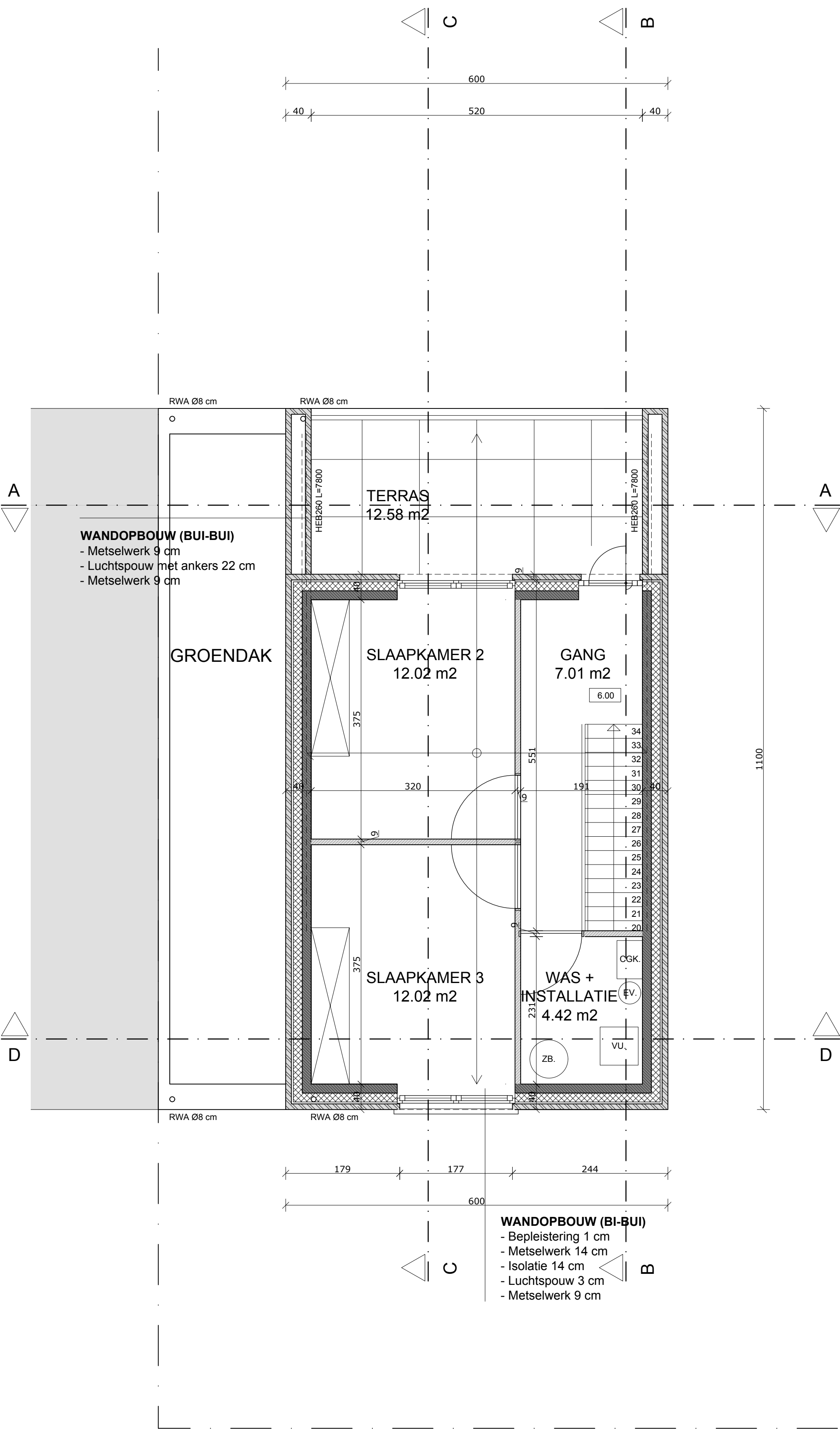
NIVEAU 2 / 1:50 35.07 m²
