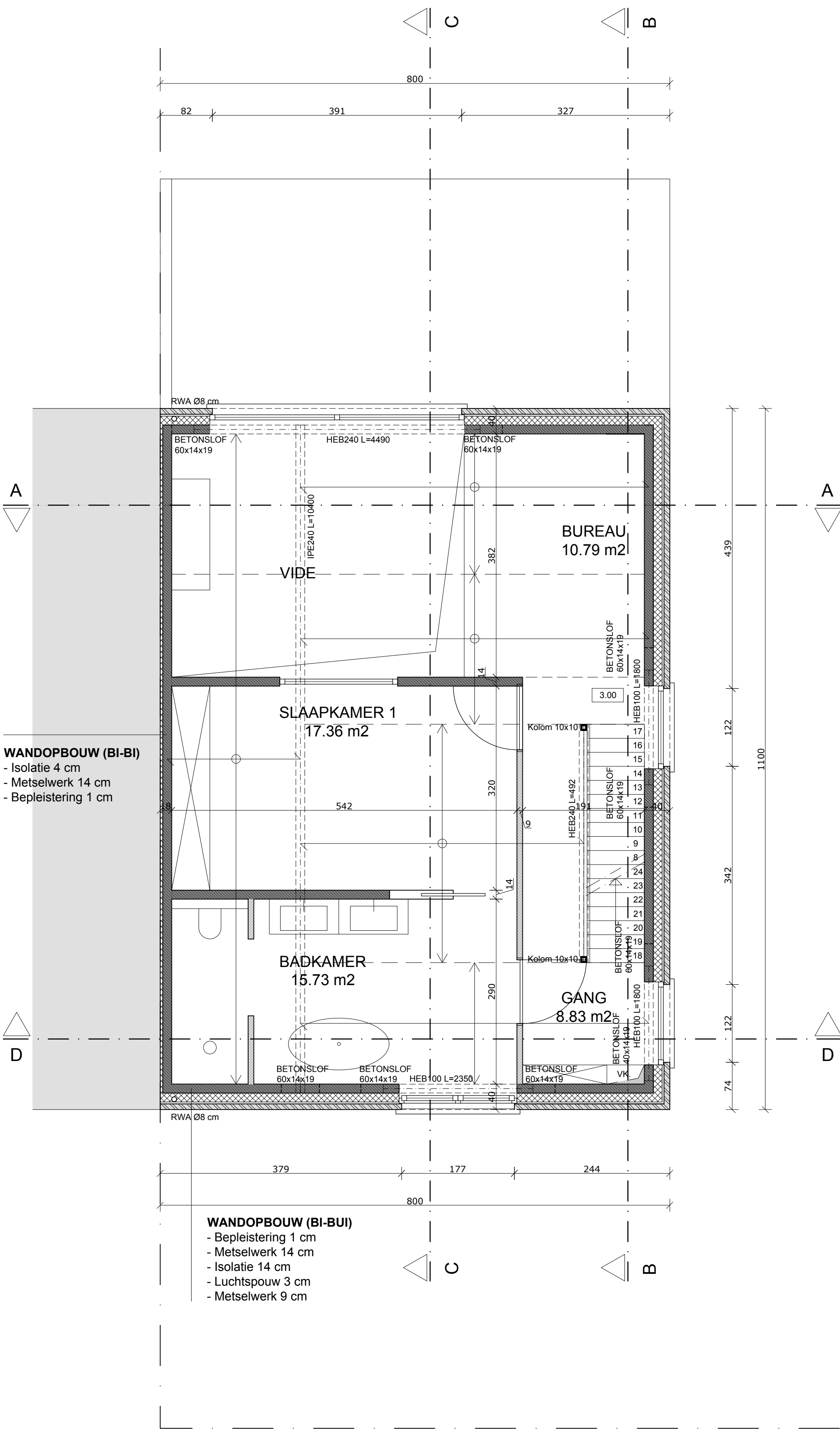
NIVEAU 1 / 1:50 52.71 m²
