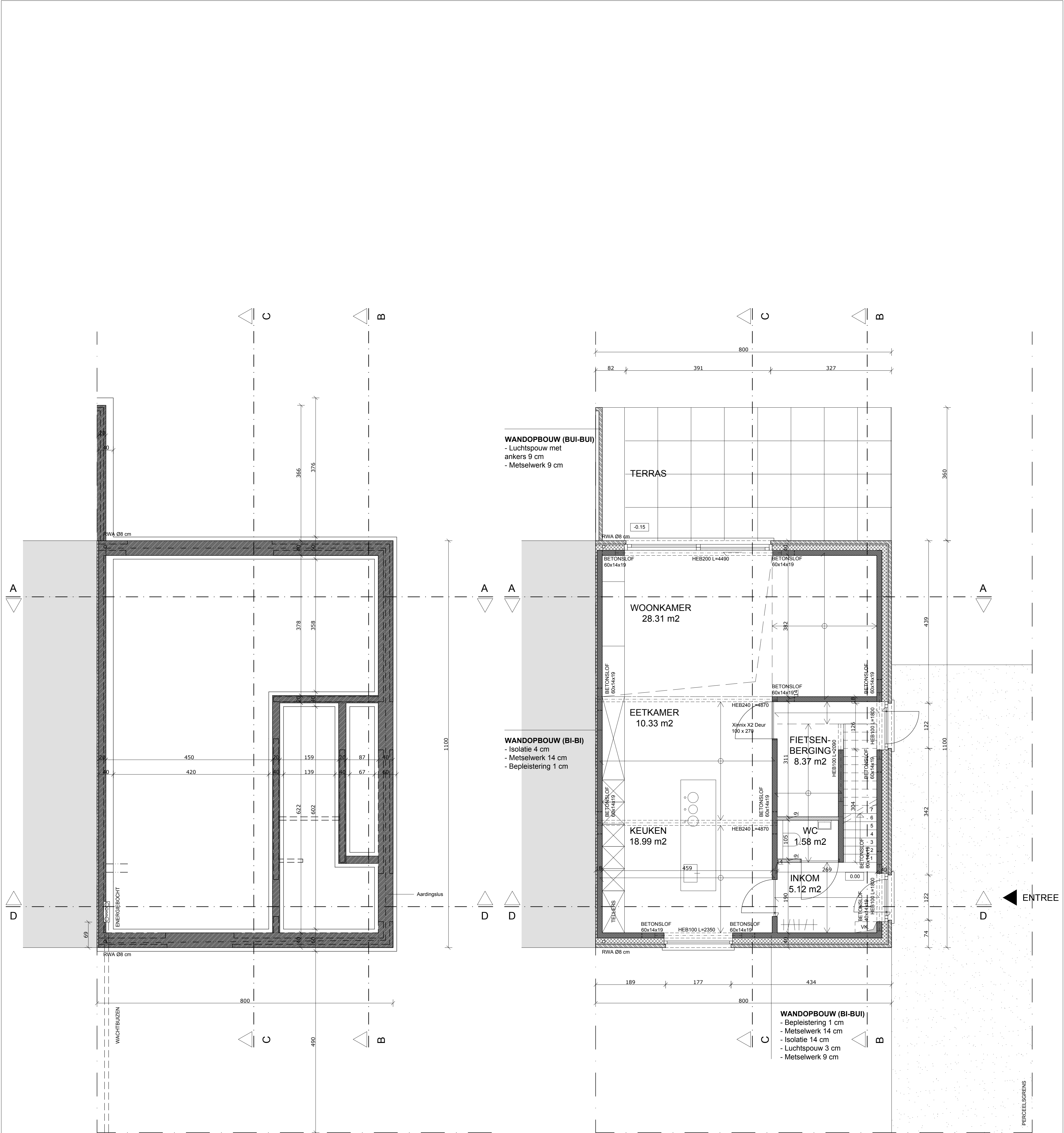
FUNDERINGSPLAN / 1:50
