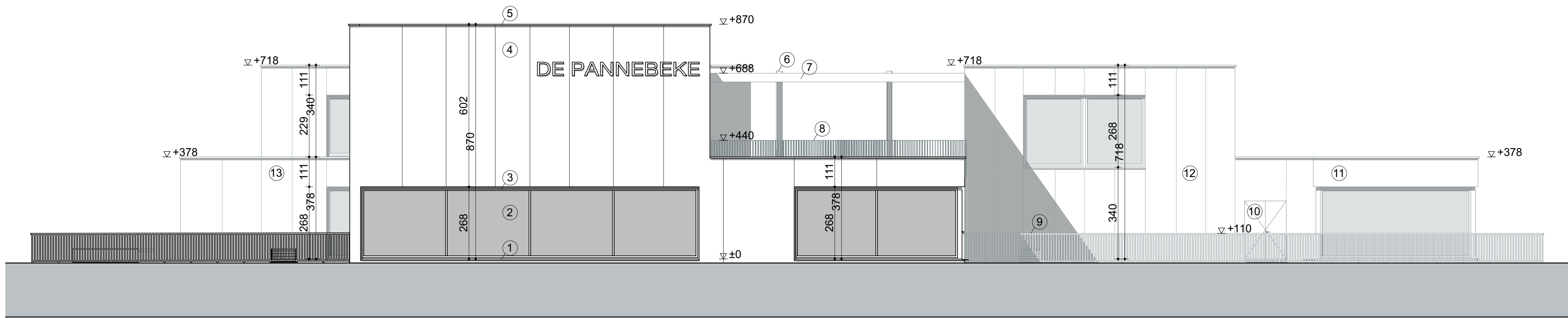
VOORGEVEL OOST / 1:100
