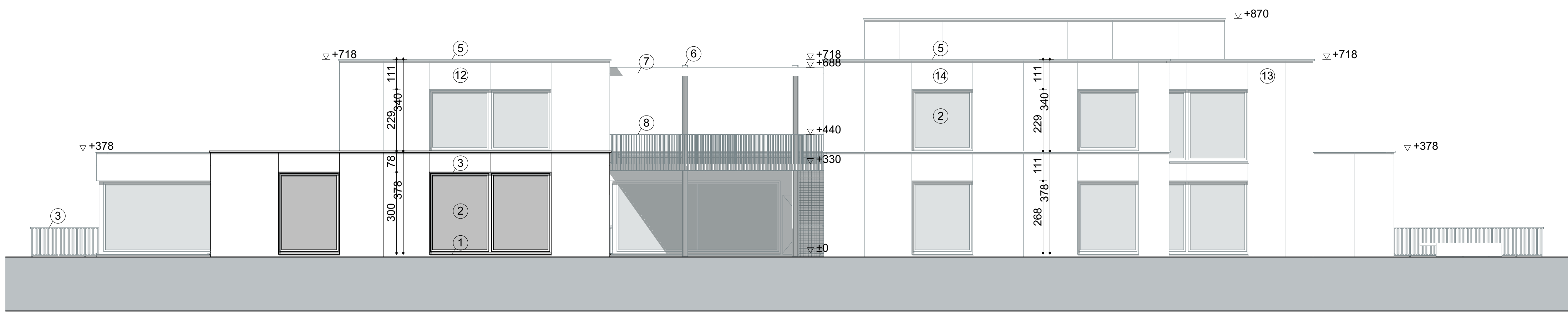
ACHTERGEVEL WEST / 1:100
